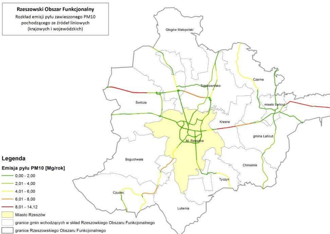
Rysunek 52. Rozkład emisji pyłu zawieszzonego PM10 pochodzącego ze źródeł liniowych (dróg krajowych i wojewódzkich) na terenie ROF 124
