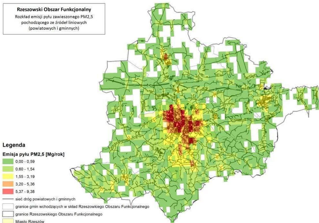
Rysunek 55. Rozkład emisji pyłu zawieszonego PM 2,5 pochodzącego ze źródeł liniowych (dróg powiatowych i gminnych) na terenie ROF 126
