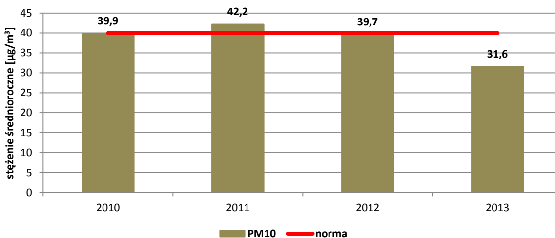
Rysunek 5. Stężenia średnioroczne pyłu zawieszonoego PM10 na przestrzeni lat 2010-2013, na stacji pomiarowej Rzeszów – ul. Szopena i Rzeszów – osiedle Nowe Miasto 41
