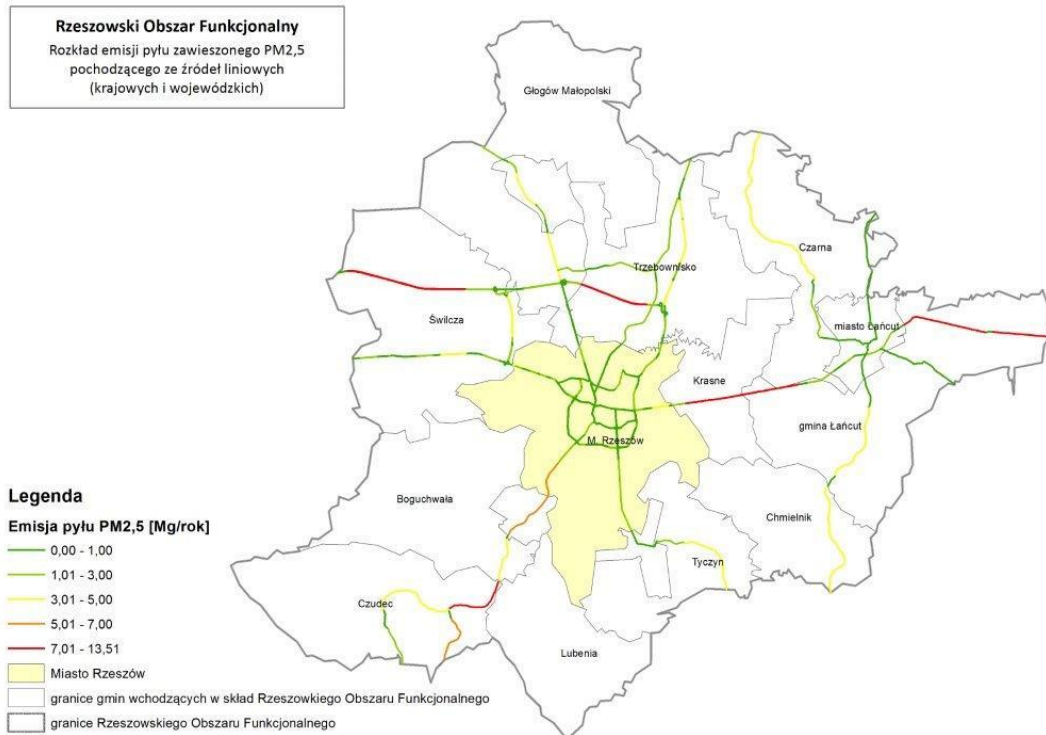
Rysunek 54. Rozkład emisji pyłu zawieszonego PM 2,5 pochodzącego ze źródeł liniowych (dróg krajowych i wojewódzkich) na terenie ROF 125
