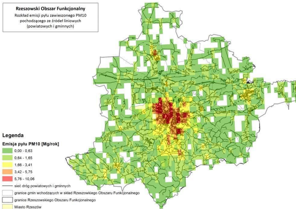
Rysunek 53. Rozkład emisji pyłu zawieszzonego PM10 pochodzącego ze źródeł liniowych (dróg powiatowych i gminnych) na terenie ROF 125
